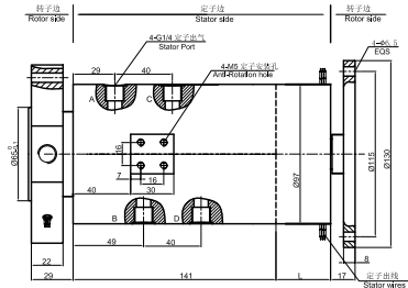
DAIPH400W-03 尺寸图
