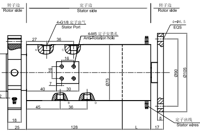
DAIPH400W-03 尺寸图
