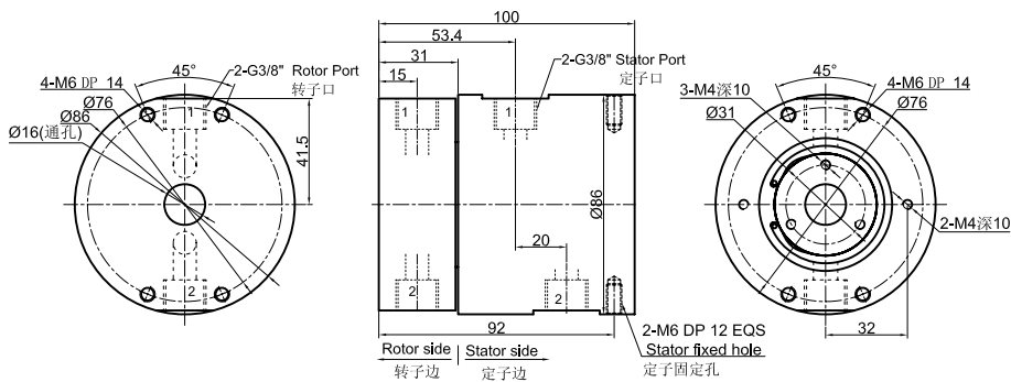
DK23 (纯气动旋转接头) 尺寸图 2进2出G3/8"牙
