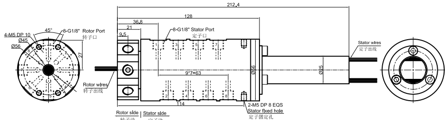
DK81S-S56 尺寸图 8进8出G1/8"牙
