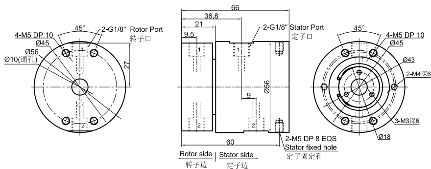
Dk21 (纯气动旋转接头) 尺寸图 2进2出G1/8"牙
