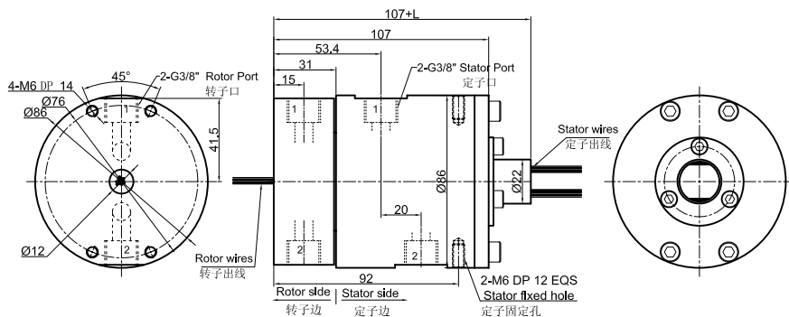
DK23S-S12(S18,S24,S36) 尺寸图 2进2出G3/8"牙+12~36路信号(2A)
