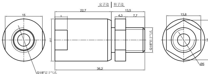
DK11A 尺寸图
