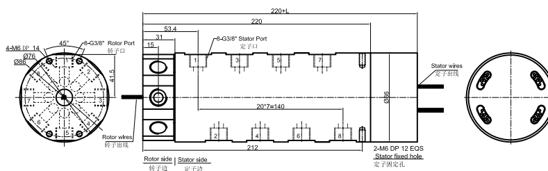
DK83-DT2586 尺寸图 8进8出G3/8"牙+信号(5A、10A)
