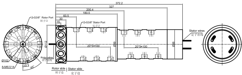
DK123-DT2586 尺寸图 12进12出G3/8"牙+信号(5A、10A)
