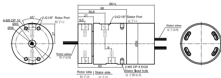
DK21-PXX-SXX 尺寸图, 2进2出G1/8牙 + 信号 (5A) /10A
