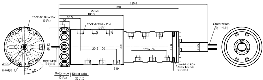
DK123S-S56 尺寸图 12进12出G3/8"牙
