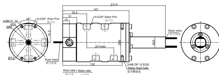
DK43S-S56 尺寸图 4进4出G3/8"牙
