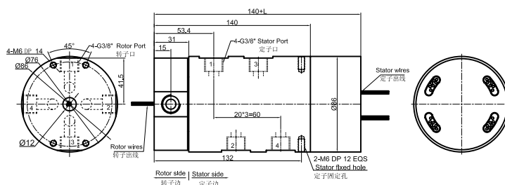
DK43-DT2586 尺寸图 4进4出G3/8"牙+信号(5A、10A)
