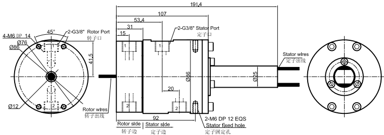
DK23S-S56 尺寸图 2进2出G3/8"牙
