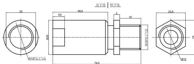
DK14A 尺寸图
