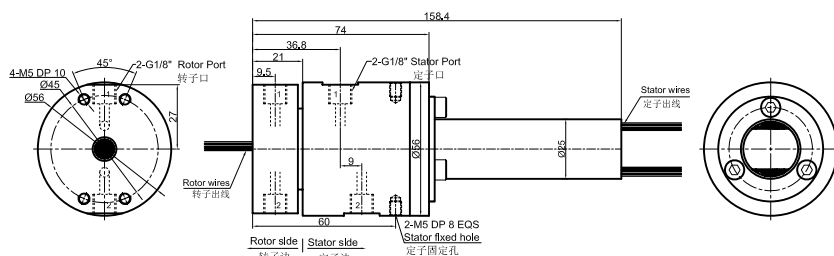
DK21S-S56 尺寸图 2进2出G1/8"牙
