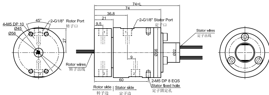
DK21S-S12(S18,S24,S36) 尺寸图 2进2出G1/8"牙+12~36路信号(2A)
