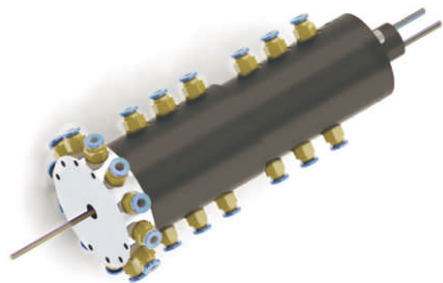
DK123 (纯气动旋转接头) 尺寸图 12进12出G3/8"牙
