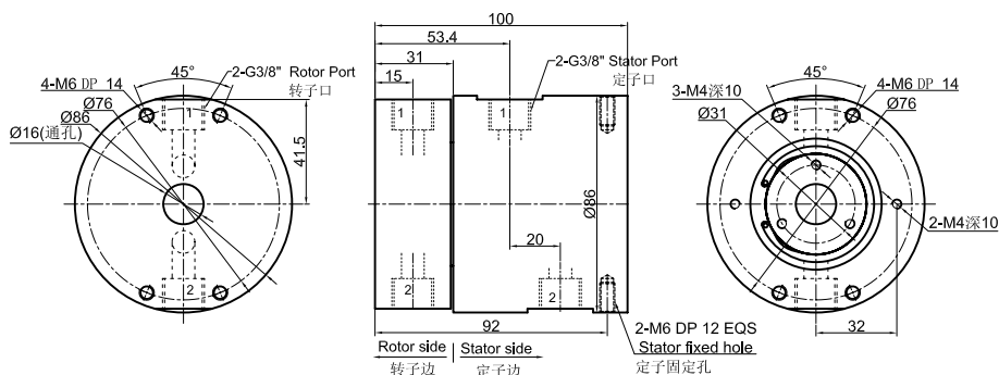
DK23 (纯气动旋转接头) 尺寸图 2进2出G3/8"牙
