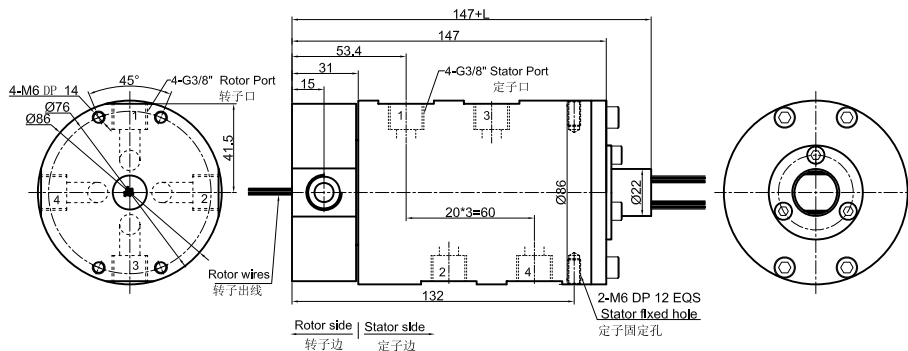
DK43S-S12(S18,S24,S36) 尺寸图 4进4出G3/8"牙+12~36路信号(2A)
