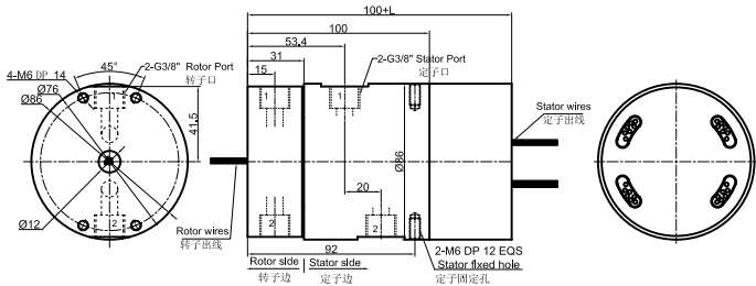
DK23-DT2586 尺寸图 2进2出G3/8"牙+信号(5A、10A)
