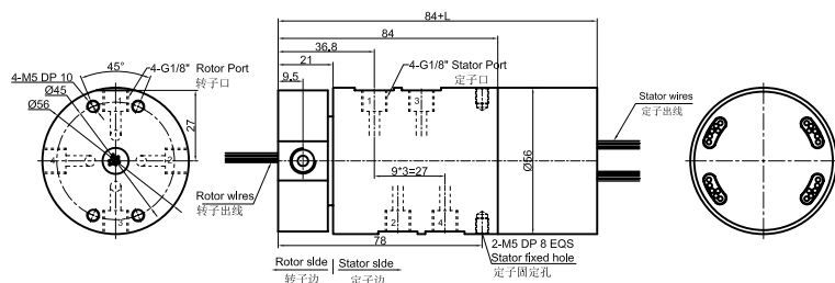
DK41-PXX-SXX 尺寸图, 4进4出G1/8牙 + 信号 (5A) /10A
