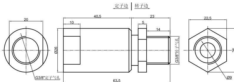
DK13A 尺寸图
