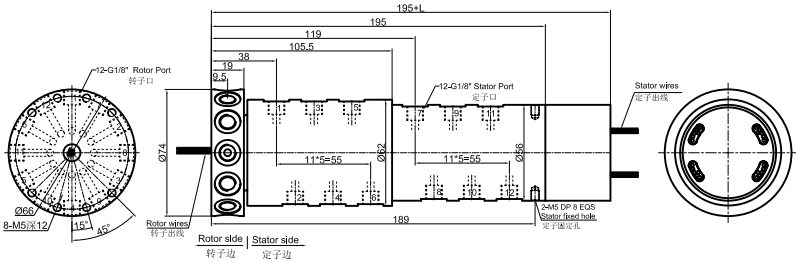
DK121-PXX-SXX 尺寸图, 12进12出G1/8牙 + 信号 ( 5A ) /10A
