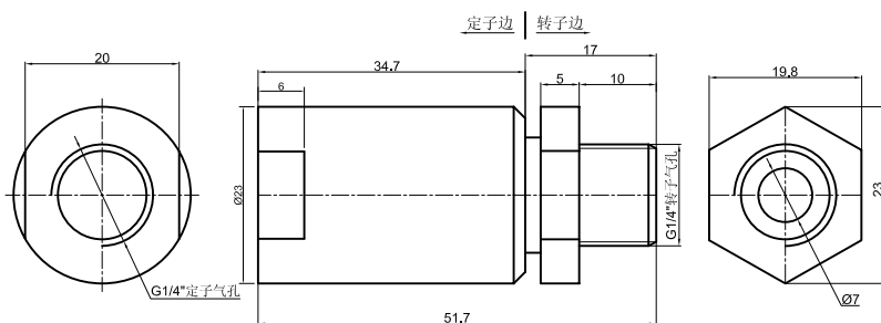
DK12A 尺寸图
