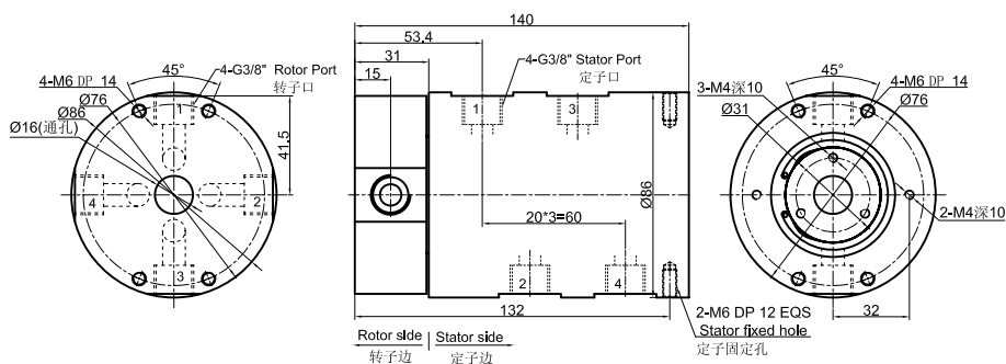
DK43 (纯气动旋转接头) 尺寸图 4进4出G3/8"牙
