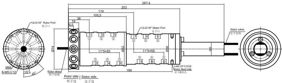
DK121S-S56 尺寸图 12进12出G1/8"牙
