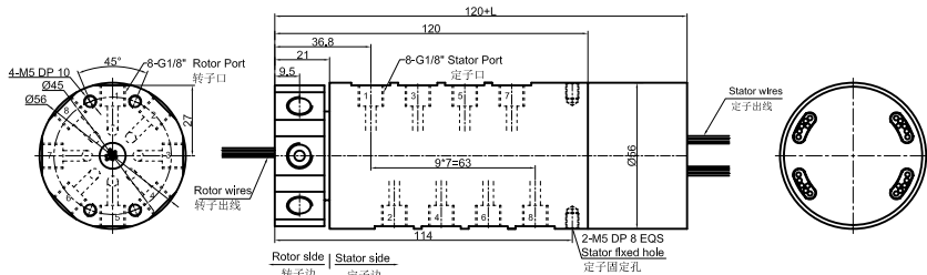
DK81-PXX-SXX 尺寸图, 8进8出G1/8牙 + 信号 ( 5A ) /10A
